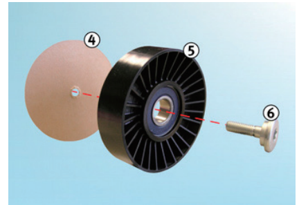
図 2：532 0138 10 - 新しい仕様
